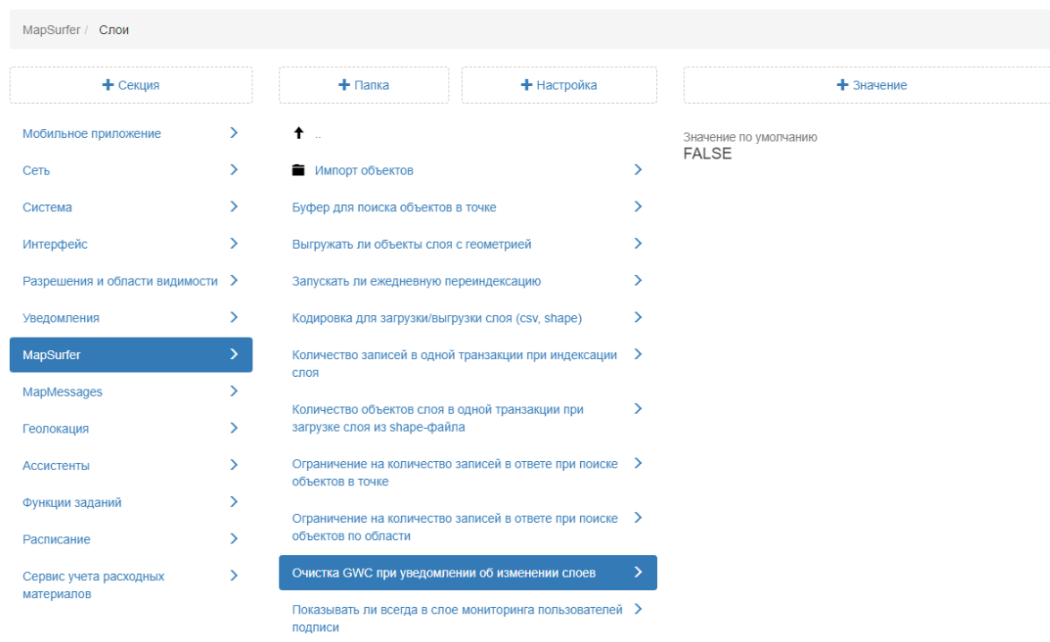
Рис. 2.223: Очистка GWC при уведомлении об изменении слоев
