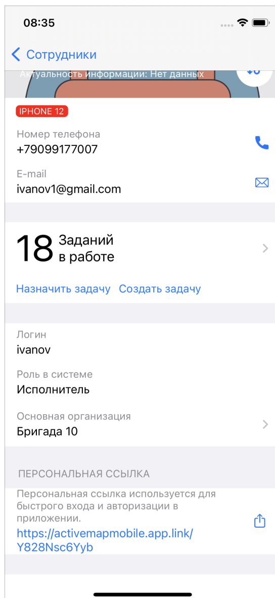
Рис. 2.36: Профиль сотрудника
