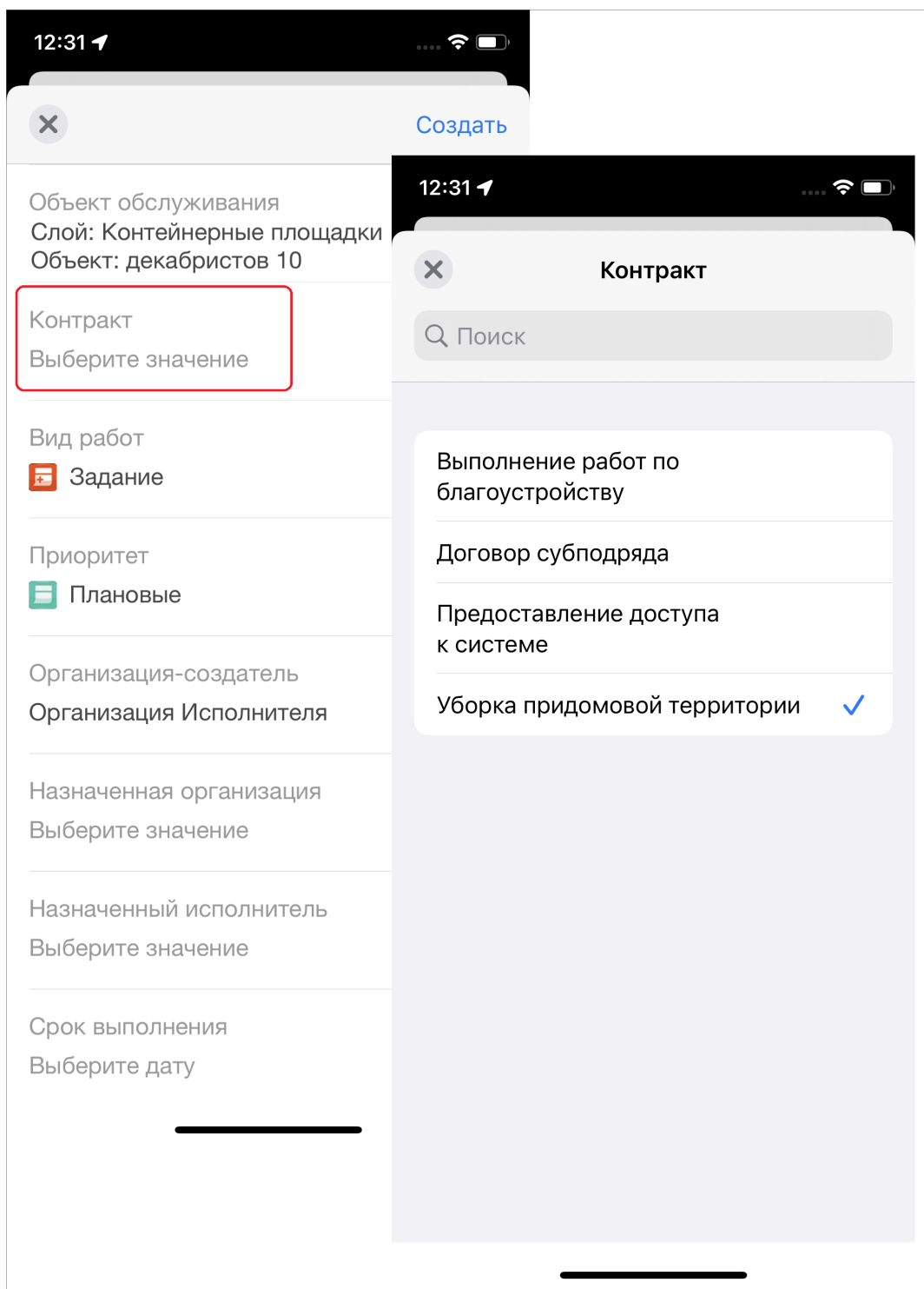
Рис. 2.23: Прикрепление контракта
