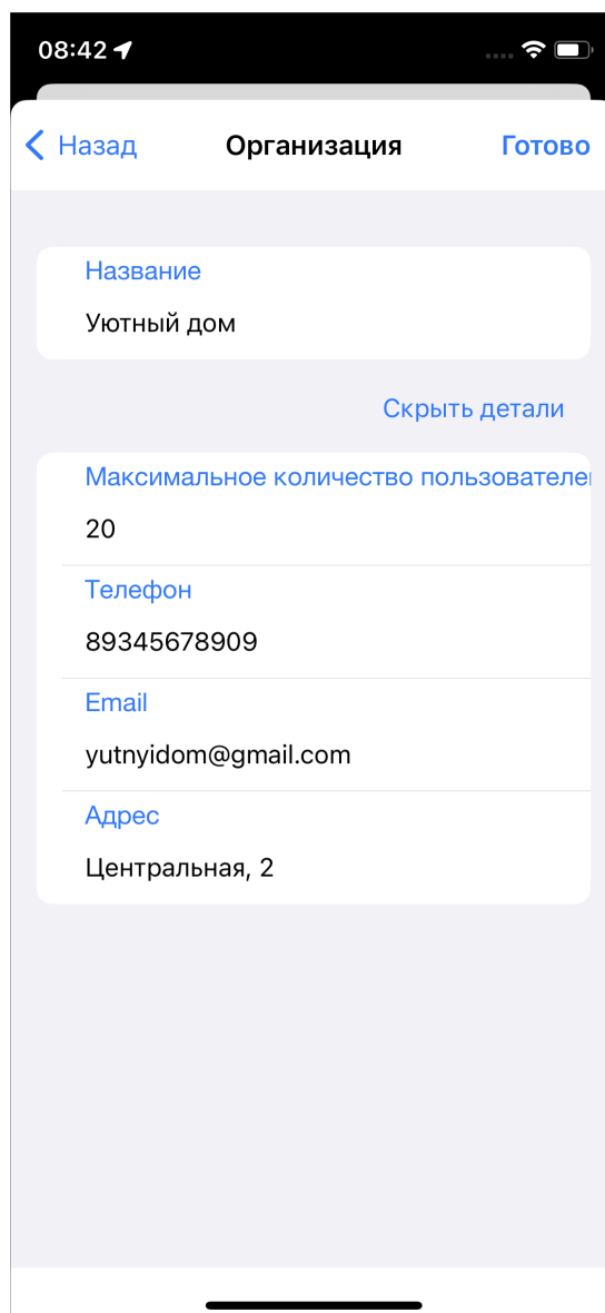
Рис. 2.44: Создание организации
