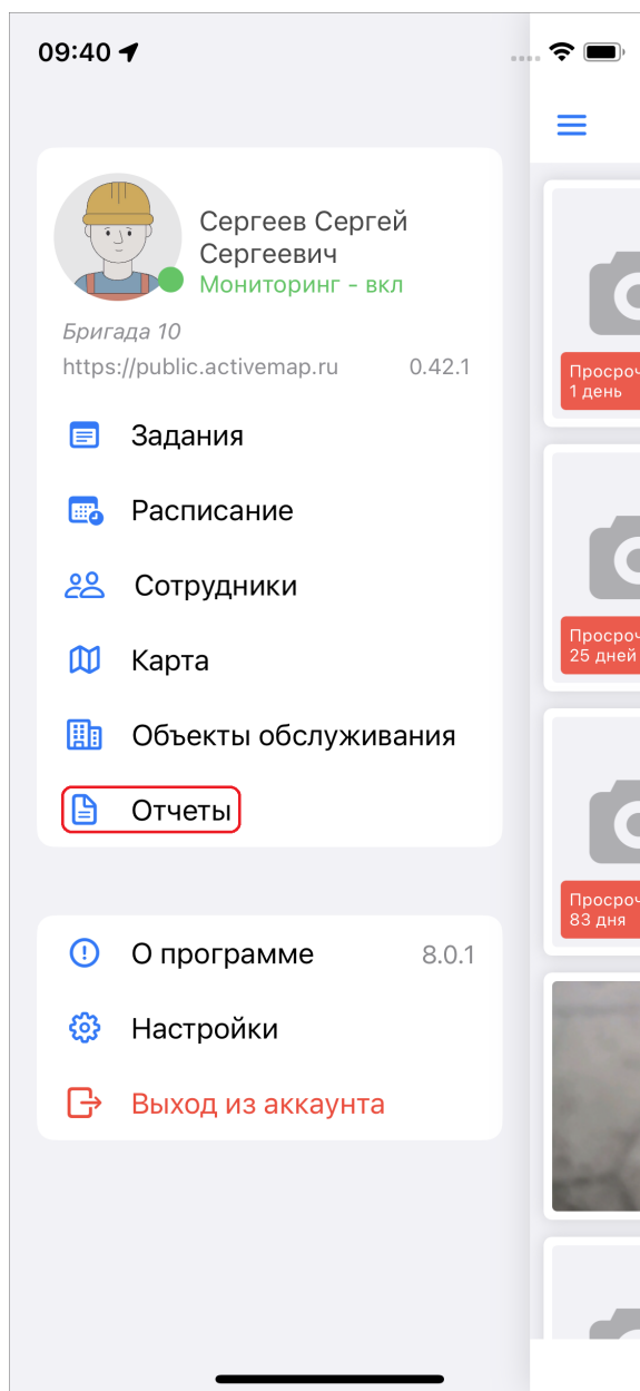
Рис. 2.84: Меню «Отчеты»
