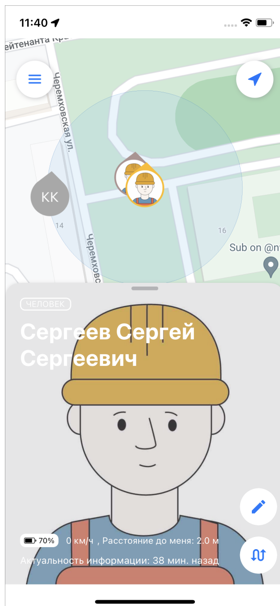
Рис. 2.75: Карточка сотрудника
