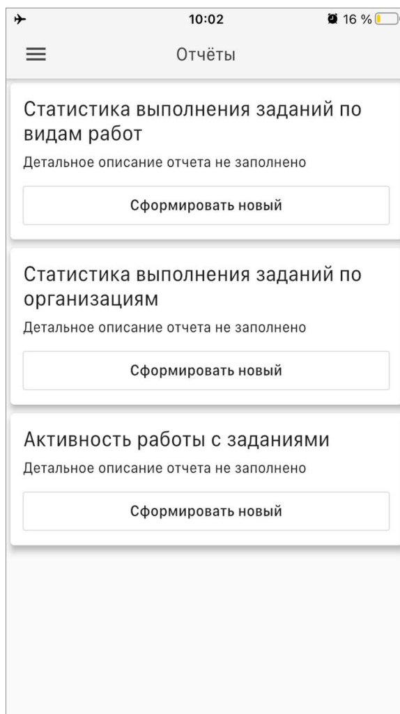
Рис. 2.85: Список отчетов
