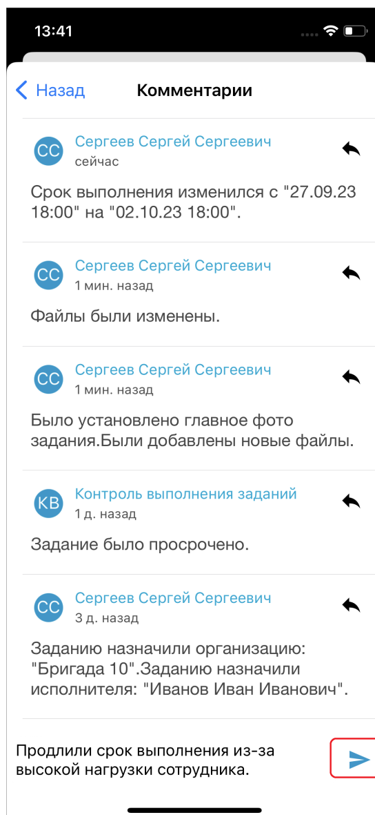
Рис. 2.32: Добавить комментарии
