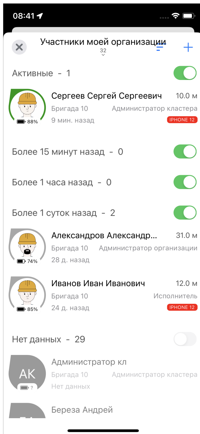
Рис. 2.73: Список пользователей
