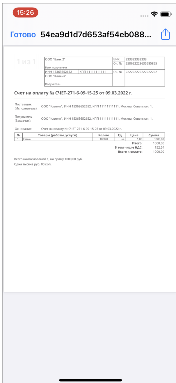
Рис. 2.91: Счет-фактура
