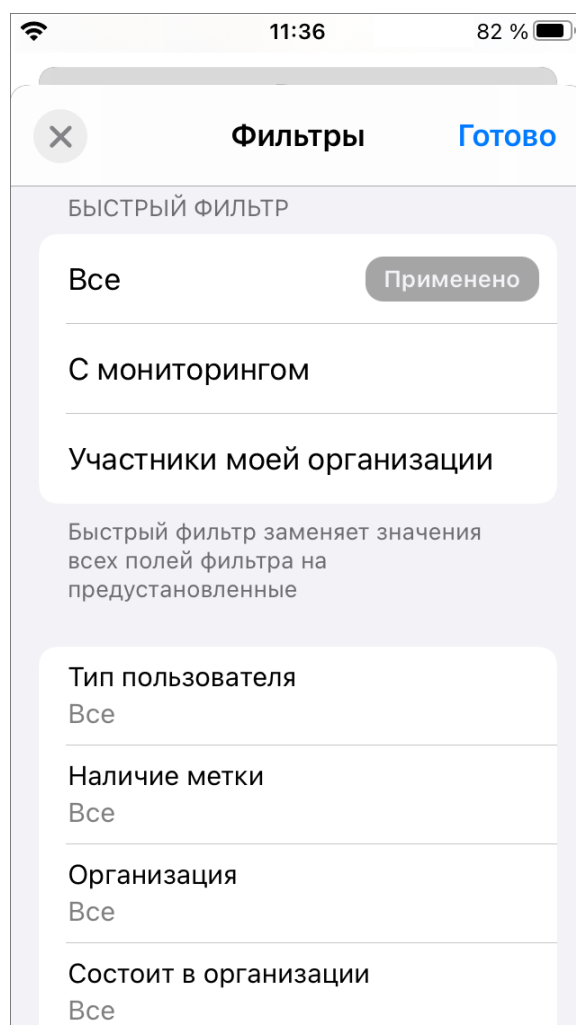
Рис. 2.74: Фильтр пользователей
