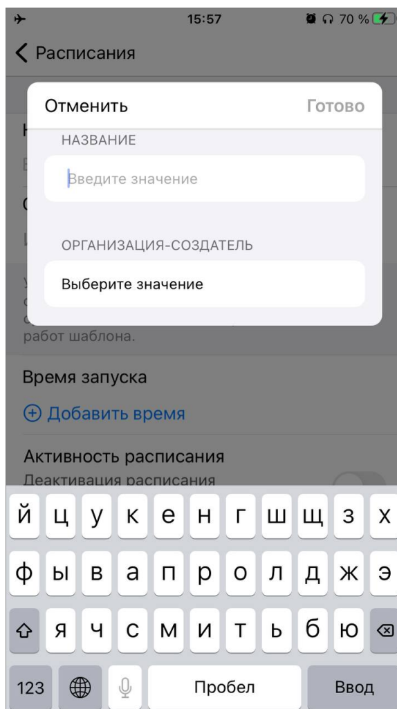
Рис. 2.81: Создание расписания
